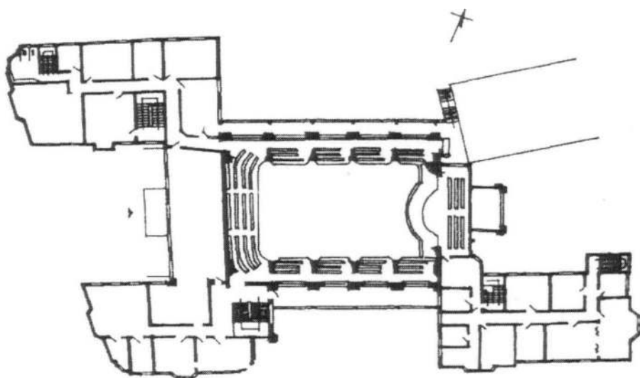
图 4.9 慕尔堂平面图
