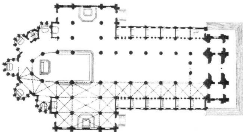
图 4.7 圣依纳爵教堂平面图
