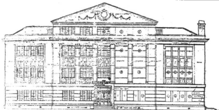
图 4.18 庚午楼正立面图（原设计图）
