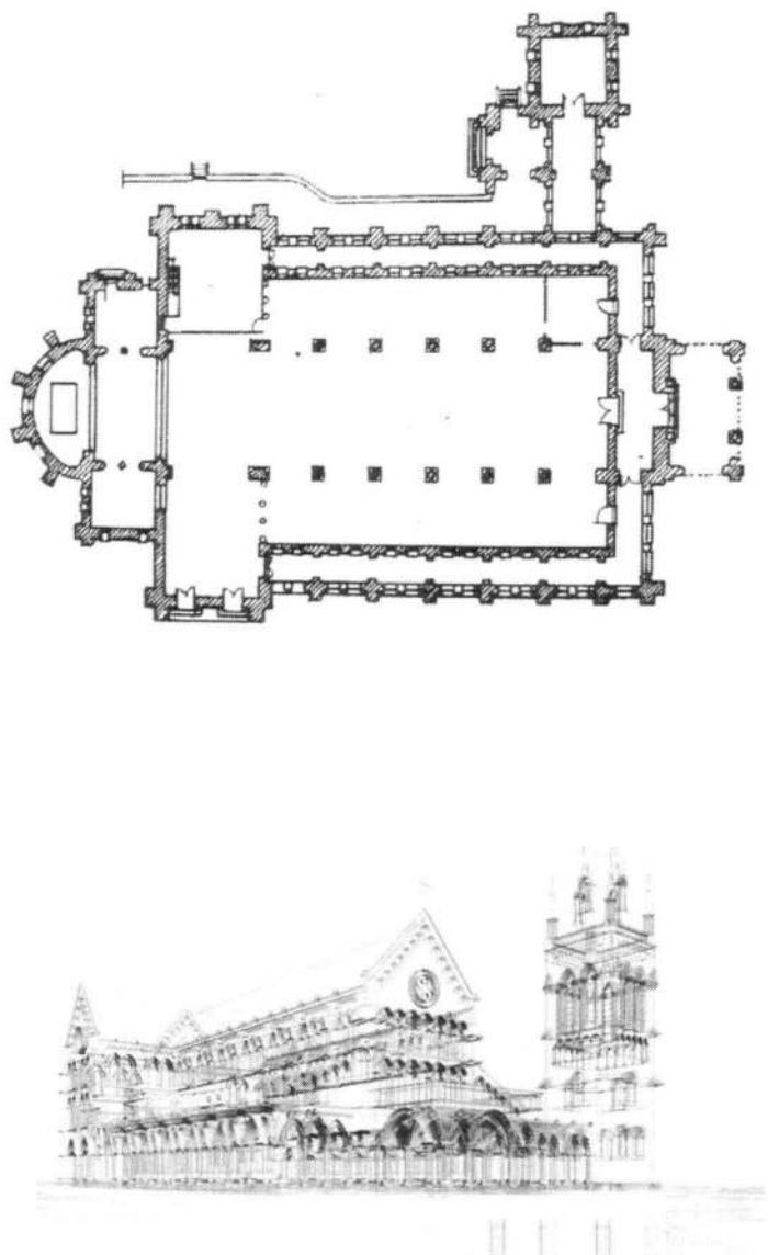
图 3.18 圣三一教堂平面和恢复模型
