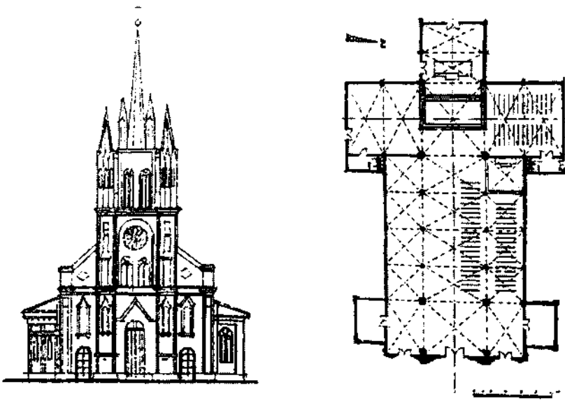
图 3.16 洋泾浜天主堂平面和立面
